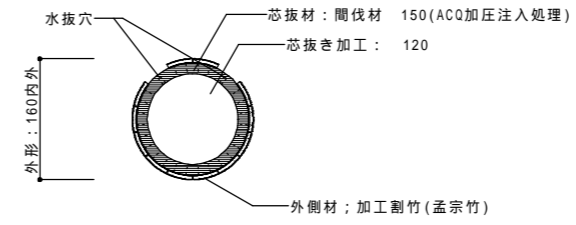
A 断面図 S = 1 : 5
