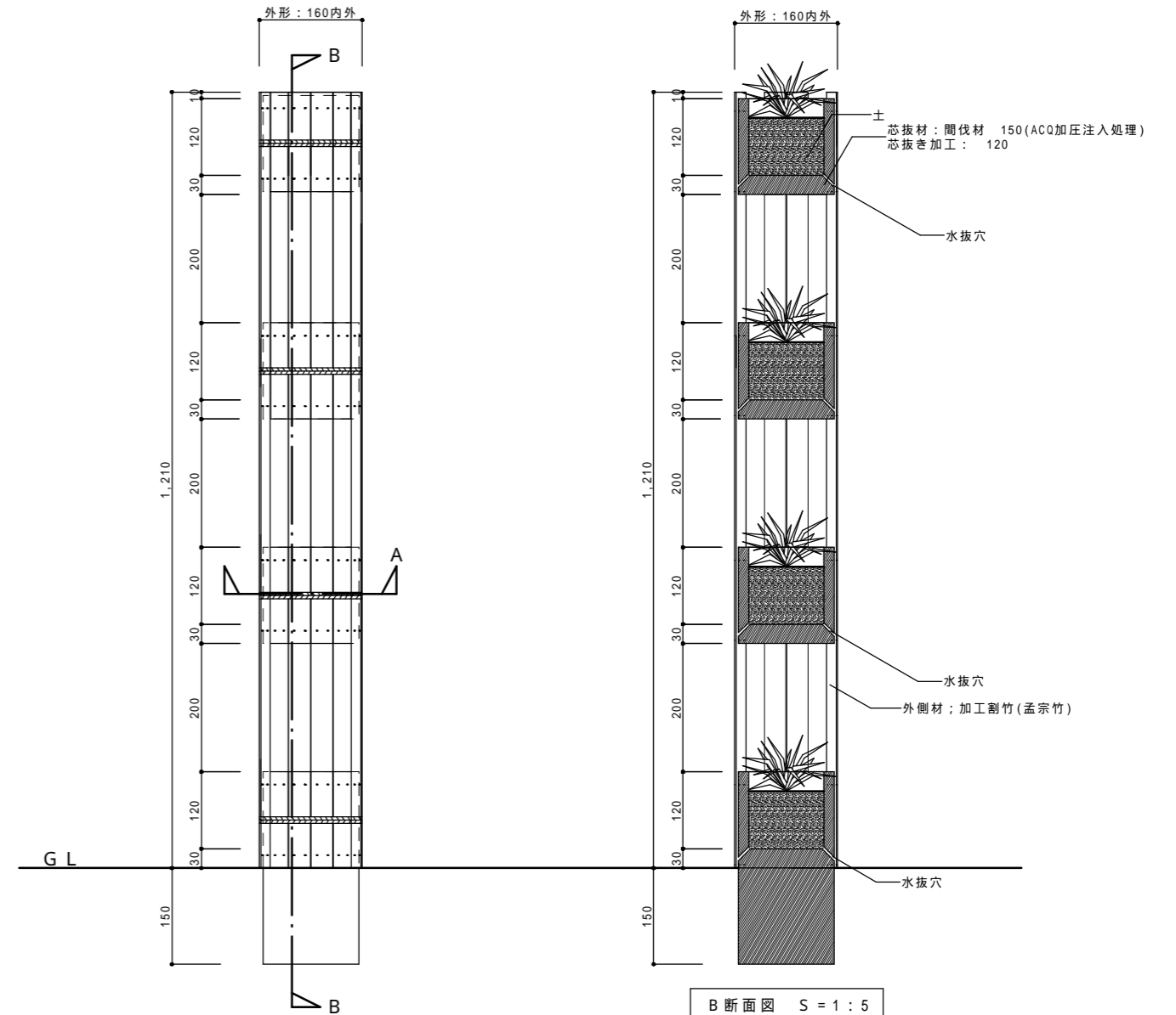
正面図 S = 1 : 5
