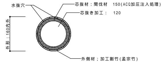
A 断面図 S = 1 : 5
