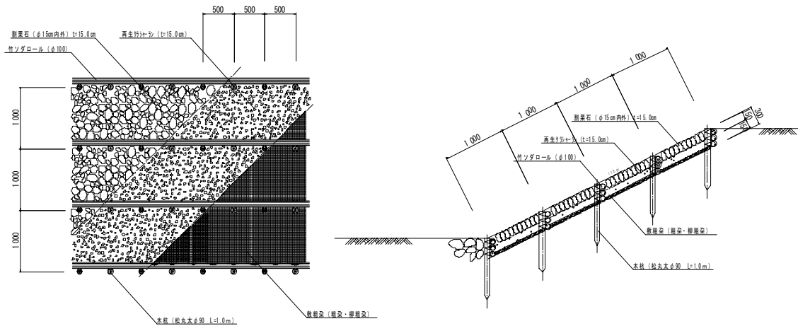
■ 竹ソダ投掛け工標準図 (1 : 2)
